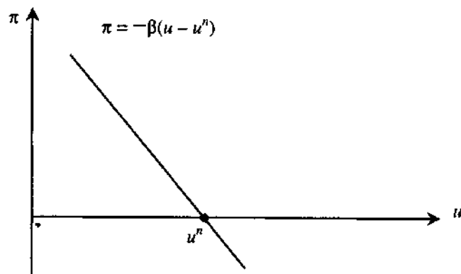
Рис. 10.4'. Кривая Филлипса
